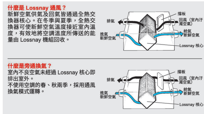
■ 自動通風模式下的旁通換氣 / Lossnay 通風分布圖
