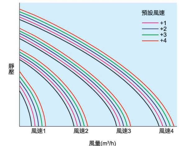
■ P-Q 曲線圖
